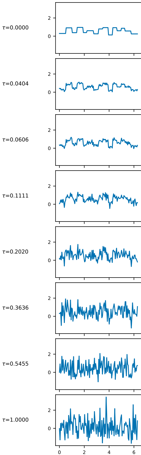
Diffusion
